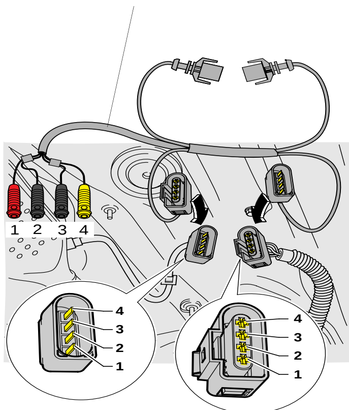
Adaptateur de sonde lambda VAS 5103
