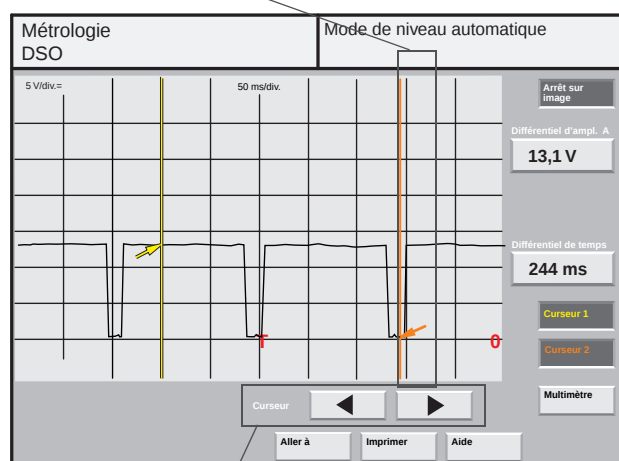
Curseur 2 avec ligne de mesure
