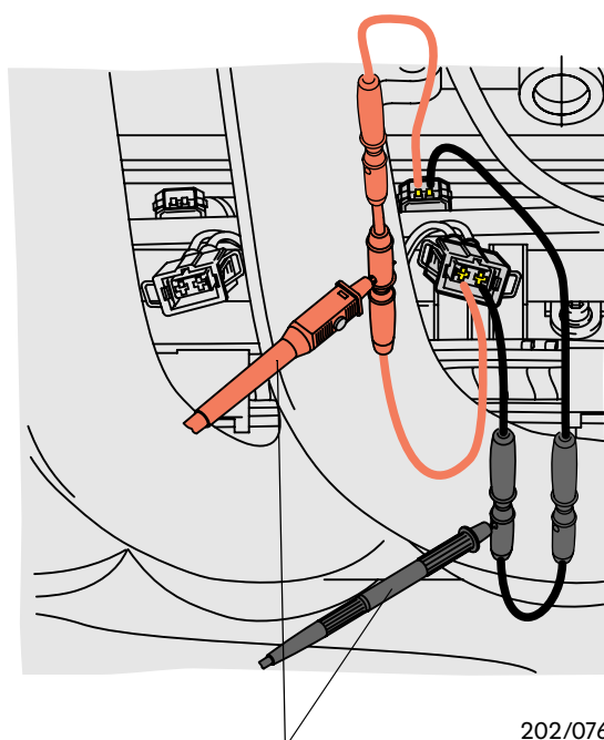
Câbles de mesure DSO
