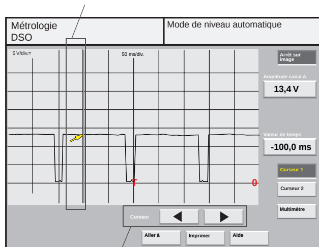
Curseur 1 avec ligne de mesure
