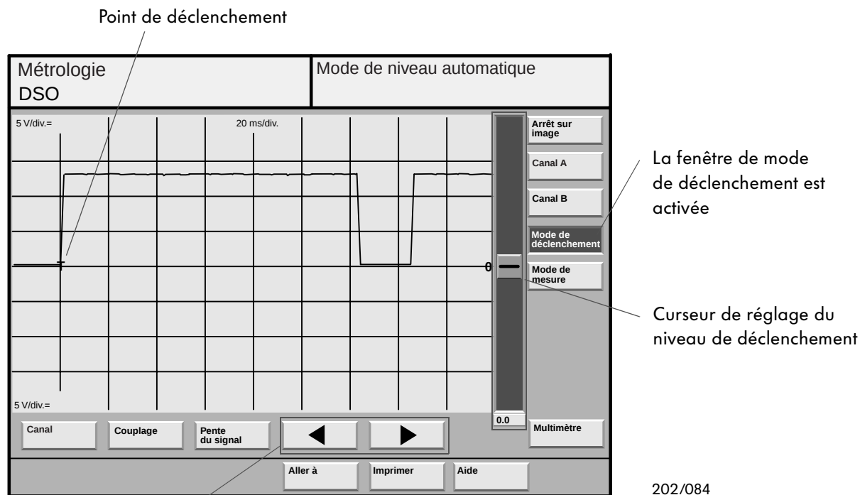
Boutons directionnels pour déplacer le point de déclenchement
