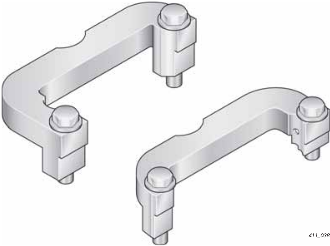
T40133/1/2 Arrêtoir pour arbre à cames
