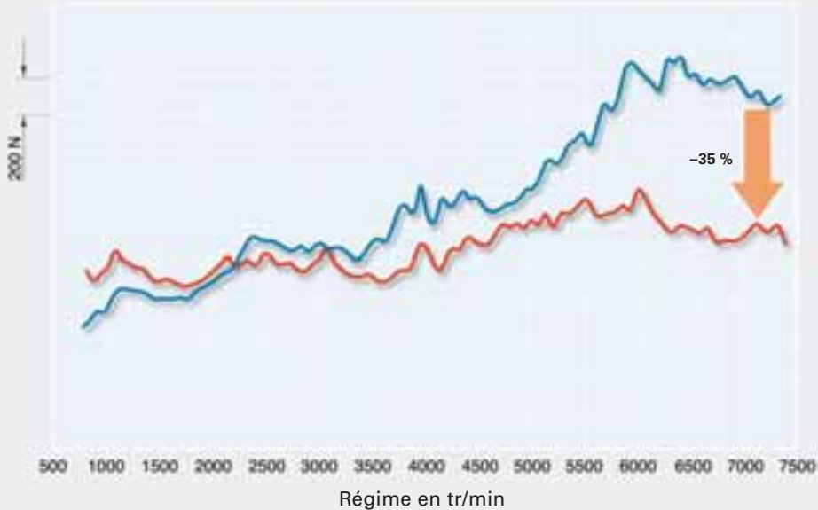
Réduction des forces exercées par la chaîne grâce à l'utilisation de pignons de chaîne triovales
