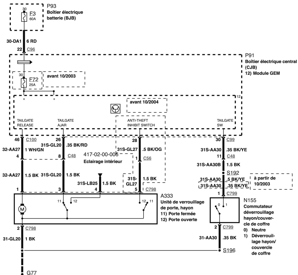
Verrouillage centralisé des portes (hayon)
