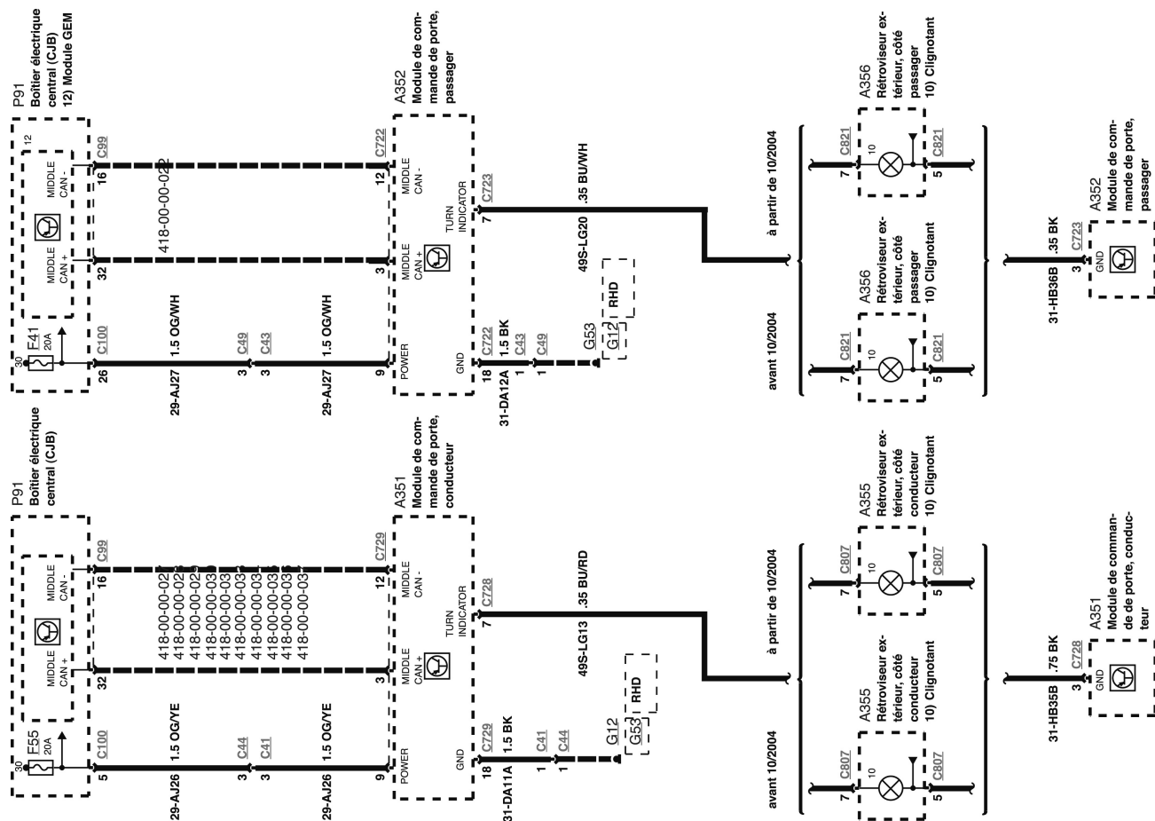
Indicateurs de direction sur les rétroviseurs
