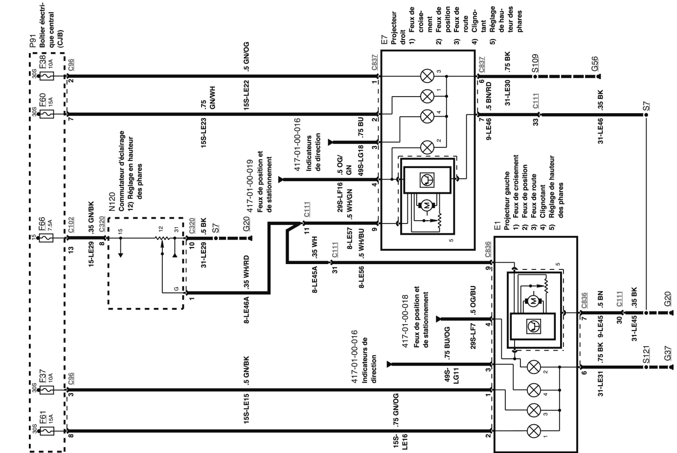
Réglage en hauteur du site des projecteurs
