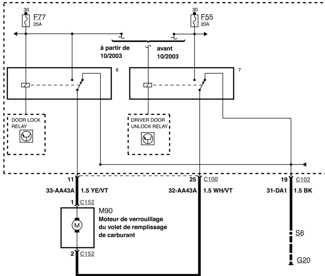
Verrouillage centralisé des portes (Trappe à carburant)
