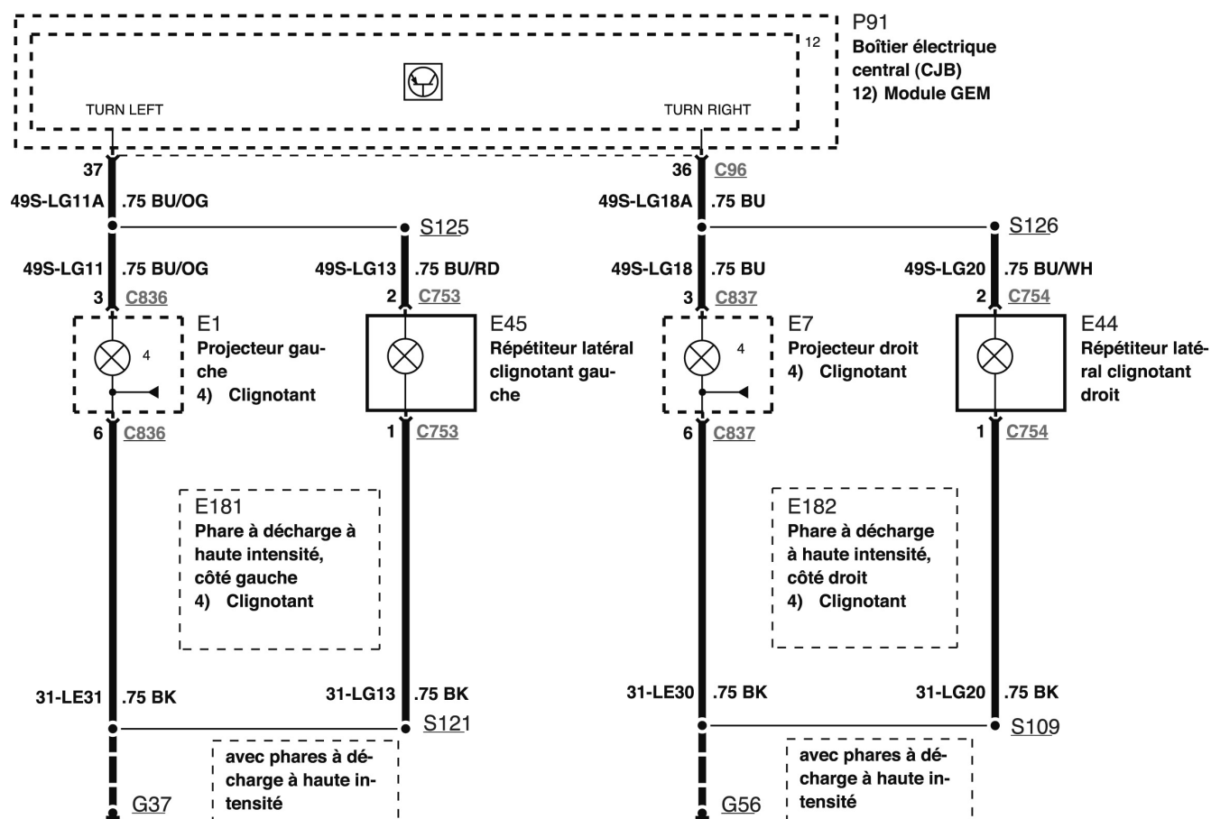
Indicateurs de direction avant et répétiteurs latéraux
