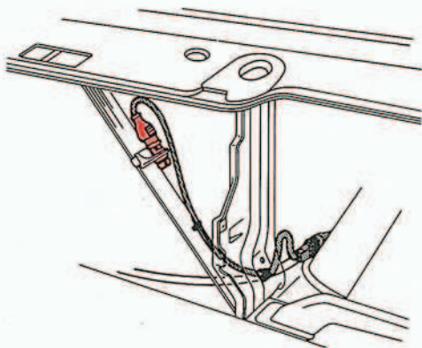
Außentemperaturgeber (G17)
