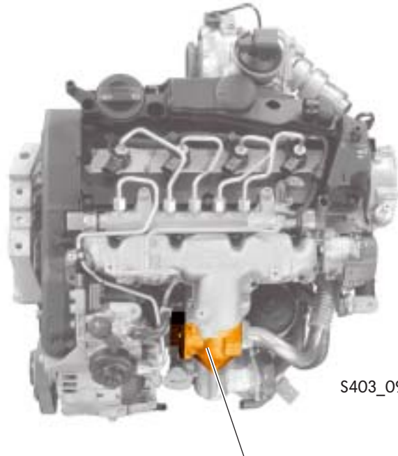
Soupape de recyclage des gaz d'échappement N18 avec potentiomètre de recyclage des gaz d'échappement G212
