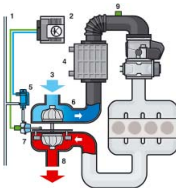
Électrovanne de limitation de la pression de suralimentation N75
