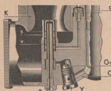
Fig. 30. — Montage 20 en coupe.
