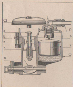
Fig. 10. — Coupe transversale du SOLEX inversé type 26 AIC (à bistarter. - Montage 21 - Ralenti à réglage d'essence).
