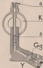
Fig. 32 — Montage 22 en coupe.
