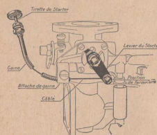
Fig. 25. — Montage de la tirette.
