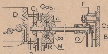
Fig. 28. — Coupe du thermostarter à membrane. Position de la bilame (B) moteur chaud : l'orifice (O) est obstrué et le clapet (C 1 ) fermé.
