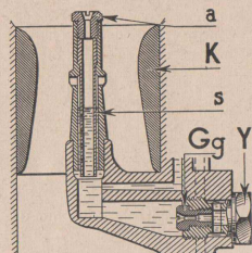
Fig. 31 — Montage 21 en coupe.
