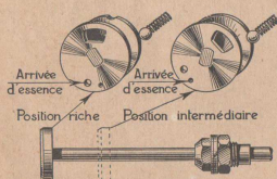
Fig. 27. — Tirette et glaces du bistarter.
