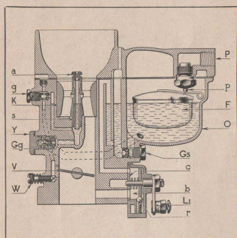
Fig. 21. — Coupe du SOLEX double-corps inversé type 30 FFIAP à bistarter, Montage 21.
